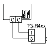
Регулирование температуры в помещении с применением устройства TG-R4XX в качестве термодатчика и задатчика
