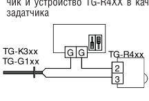
Термодатчик максимального предельного значения
